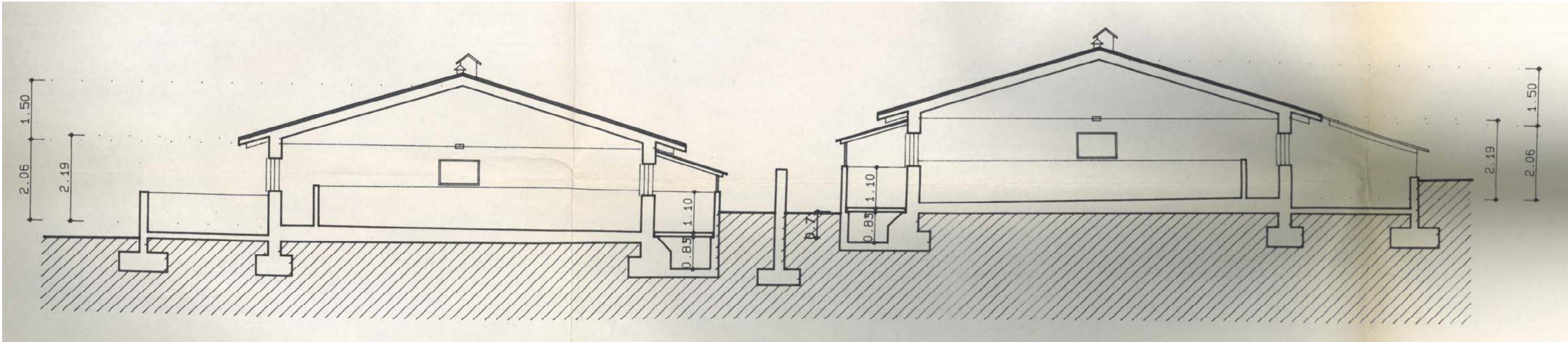
SEZIONE X-X' SCALA 1:100
